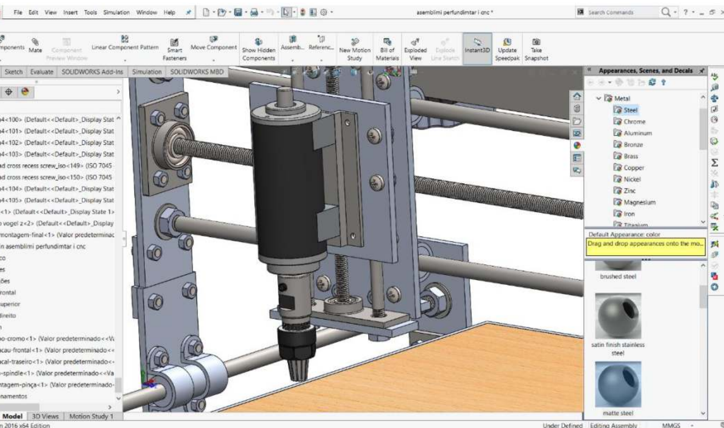
Figure 95 Dërgje 3D e shpindelit
