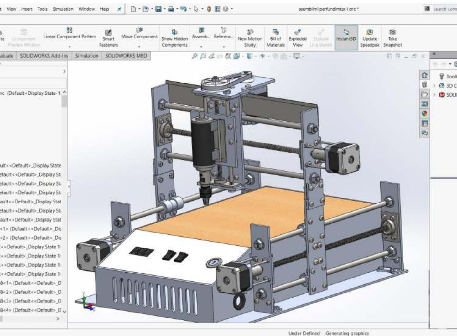
Figure 99 Të gjitha pjesët e prototipit të montuara
